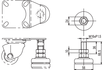
専用アジャスターフット付 HJ-50B-MC AD-50
